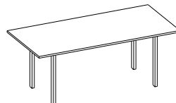
stół konferenc. DST190 FE 1900x900x740h
